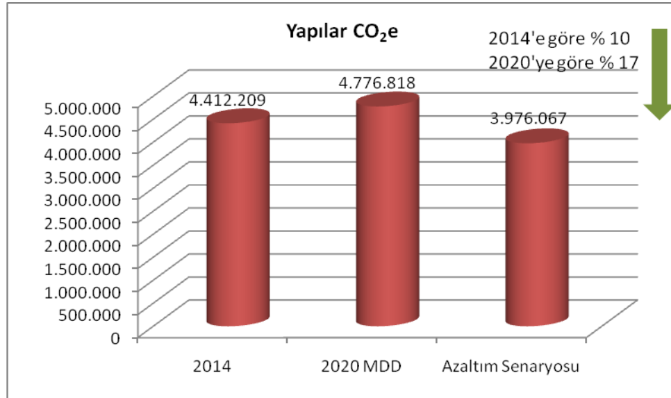
ŞEKİL 5-3: YAPILARDAN KAYNAKLANAN SALIMLARIN GELİŞİMİ.
