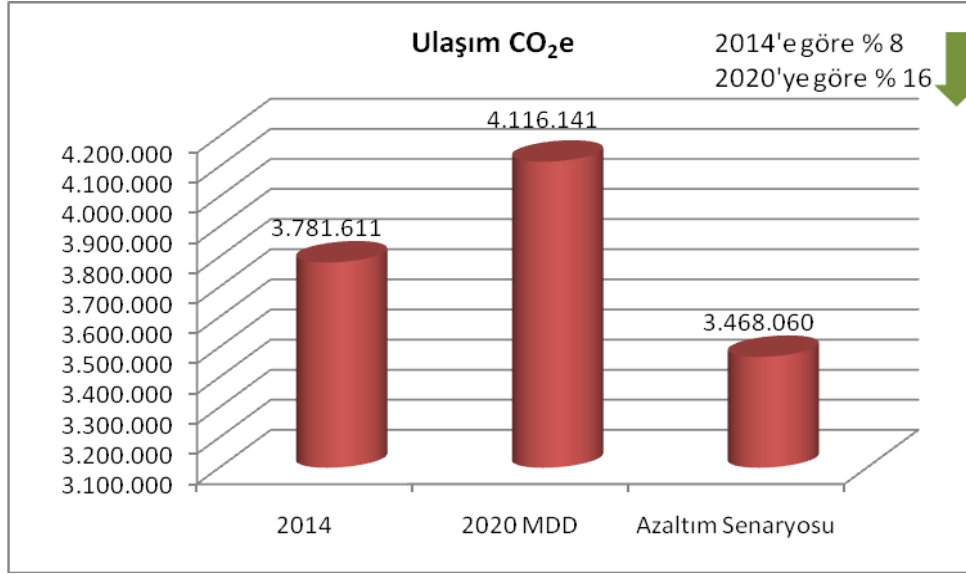
ŞEKİL 5-4: İZMİR ULAŞIM SALIMLARININ GELİŞİMİ.
