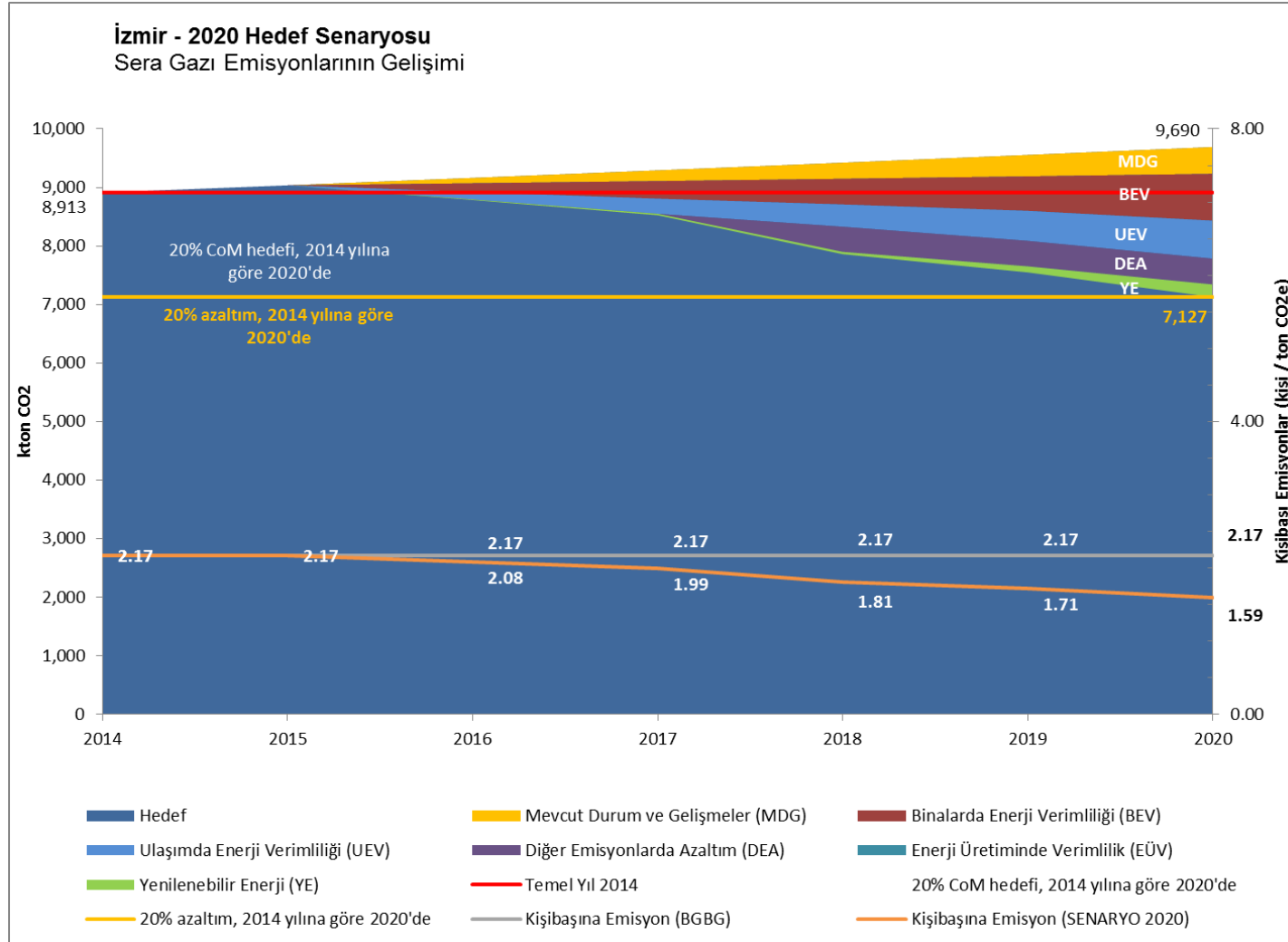
ŞEKİL 4-17: İZMİR KENTSEL SALIMLARI 2020 HEDEF SENARYOSU
