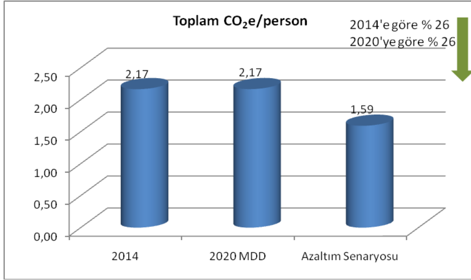
ŞEKİL 5-2: İZMİR KİŞİ BAŞI SERA GAZI SALIMLARININ DEĞİŞİMİ
