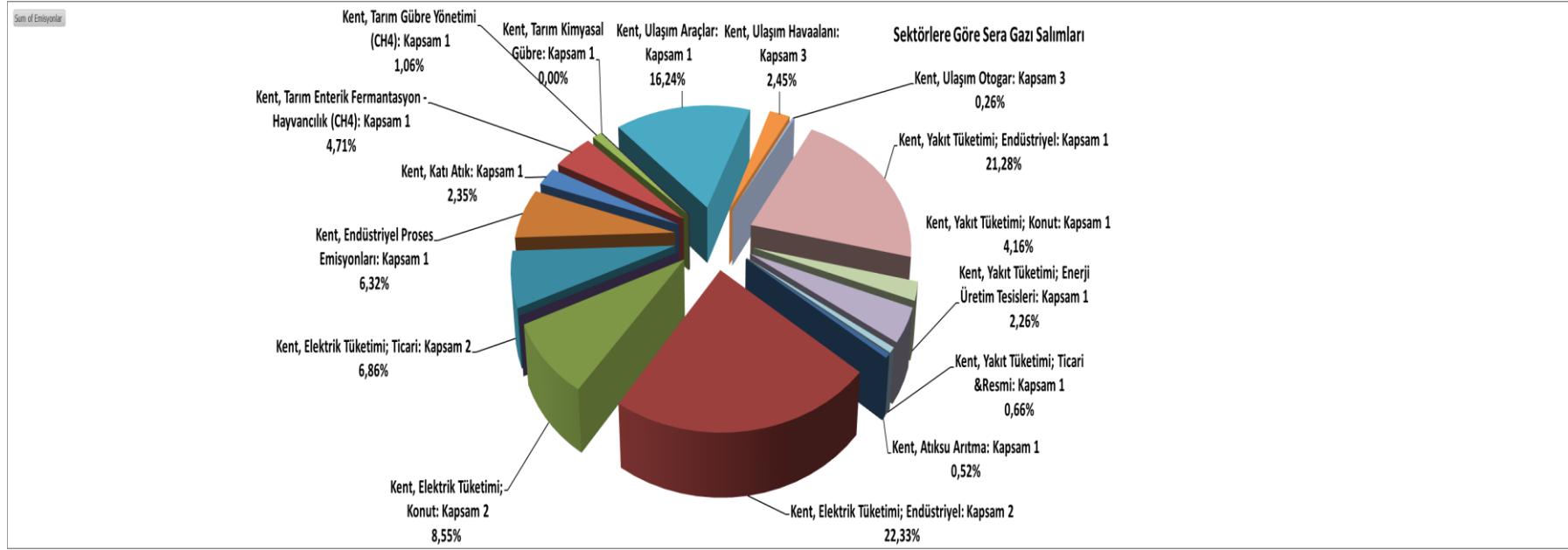
ŞEKİL 3-4: İZMİR SALIM ENVANTERİ SONUÇLARINA GÖRE SEKTÖRLERİN TOPLAM SALIMA KATKILARI
