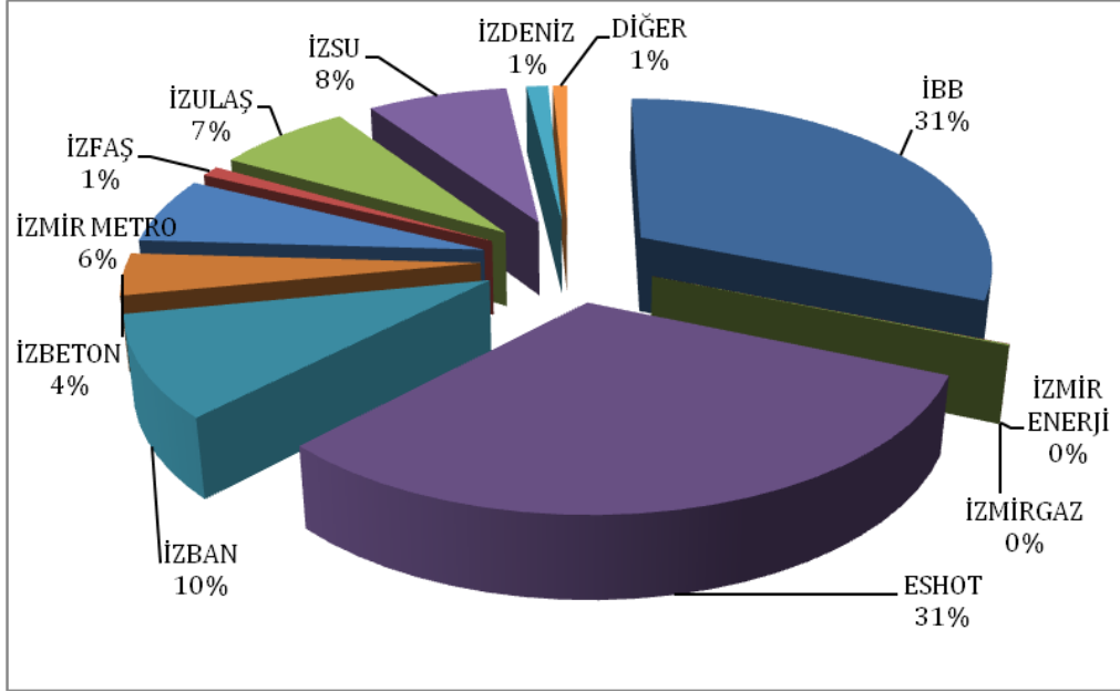
ŞEKİL 3-2: İBB KURUMSAL SERA GAZI SALIMLARININ İŞTİRAKLER BAZINDA DAĞILIMI
