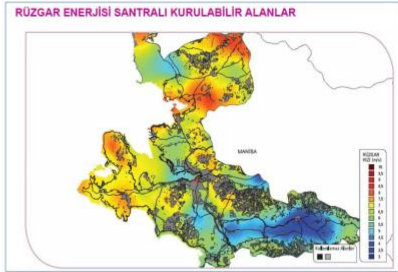
ŞEKİL 4-14: İZMİR'DE RÜZGÂR ENERJİSİ SANTRALİ KURULABİLİR ALANLAR
