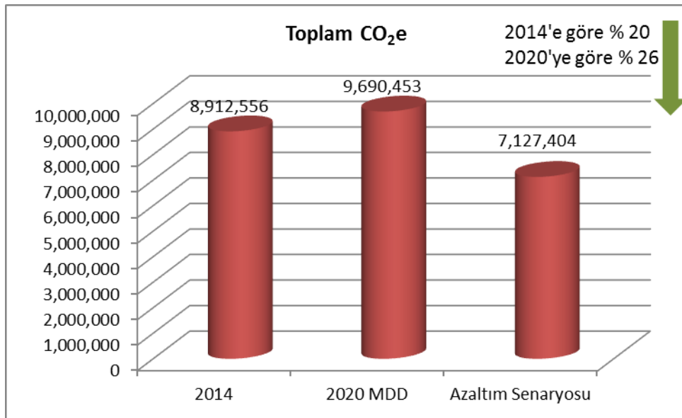
ŞEKİL 5-1: İZMİR TOPLAM SALIMLARI - MEVCUT DURUMUN DEVAMI VE AZALTIM SENARYOLARI
