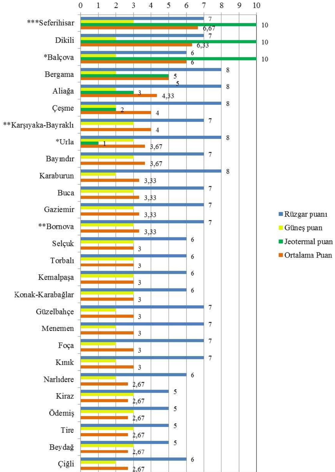
ŞEKİL 4-16: PUANLAMA YÖNTEMİNE GÖRE İZMİR'DEKİ İLÇELERİN YENİLENEBİLİR ENERJİ KAYNAKLARININ POTANSİYELİ
