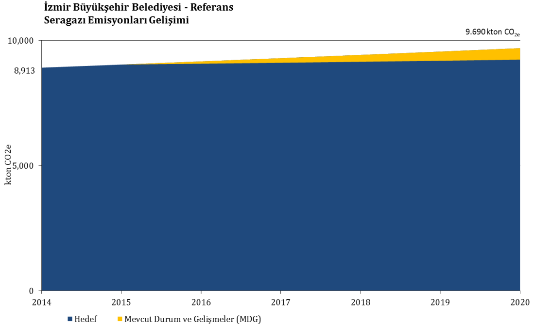
ŞEKİL 4-2: İZMİR SERA GAZI SALIM TAHMİNLERİ, 2020
