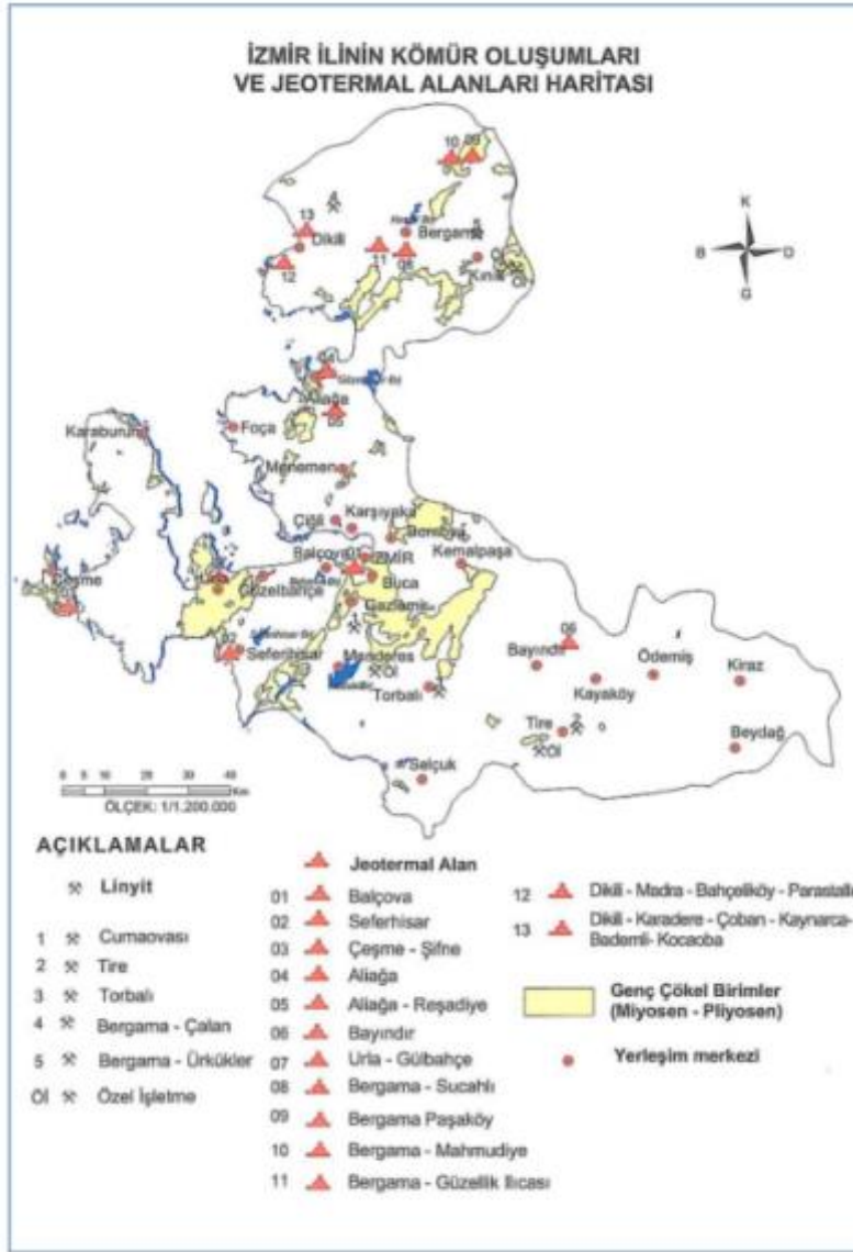
ŞEKİL 4-15: İZMİR BÖLGESİ JEOTERMAL KAYNAKLARINI GÖSTERİR HARİTA
