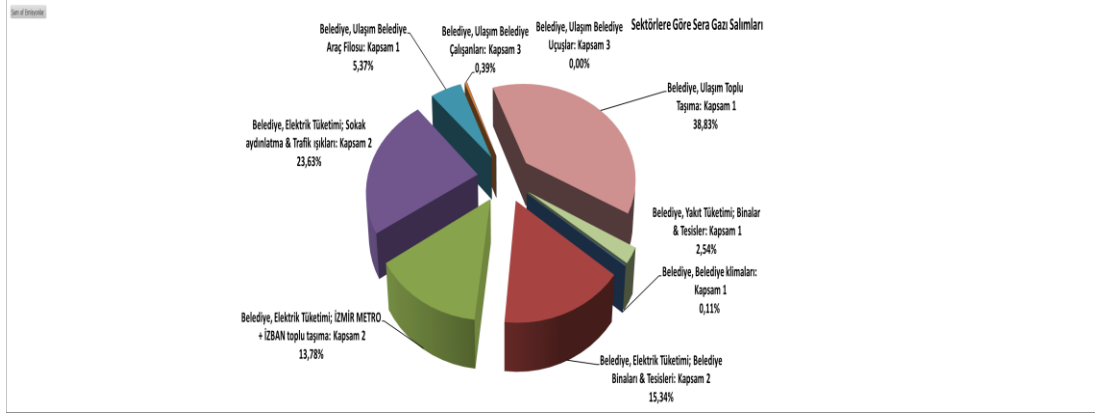
ŞEKİL 3-1: İZMİR BÜYÜKŞEHİR BELEDİYESİ KURUMSAL SERA GAZI SALIMLARININ DAĞILIM
