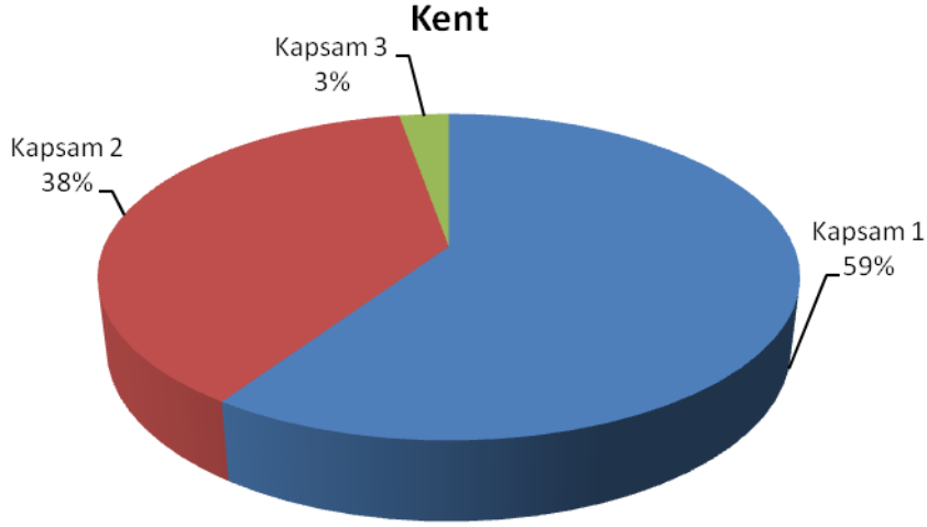
ŞEKİL 3-3: ICLEI KAPSAM TANIMLARINA GÖRE KENT SALIMLARI VE DAĞILIMI.
