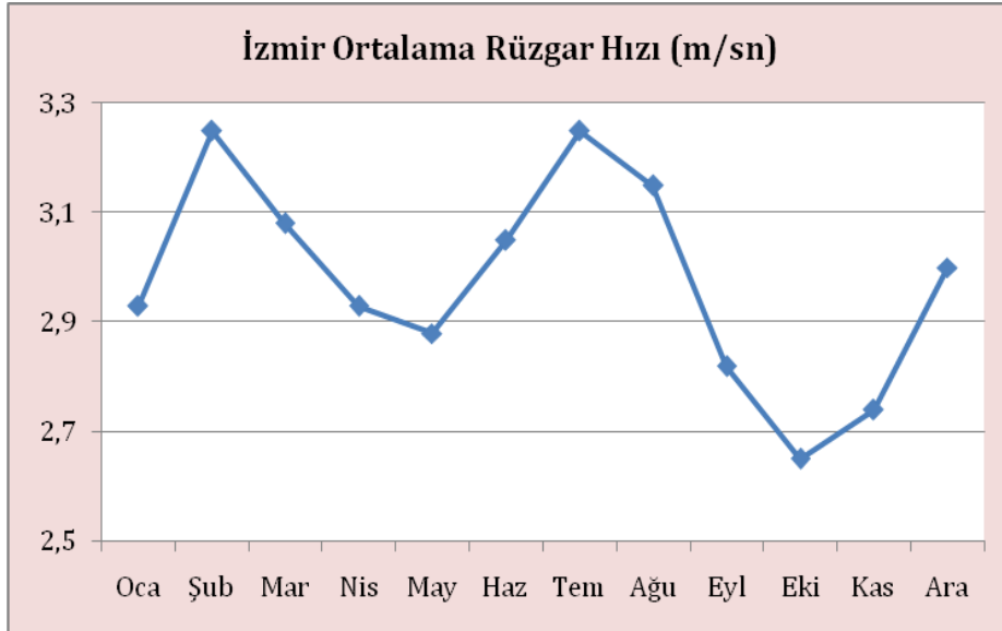
ŞEKİL 2-5: İZMİR İLİ ORTALAMA RÜZGAR HIZI
